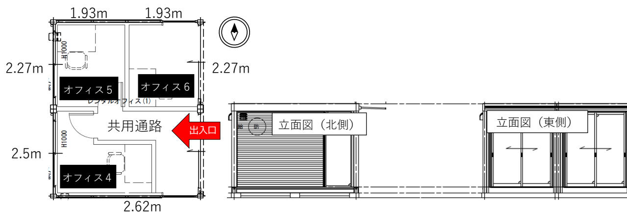
オフィス棟 C (平面図と立面図)
