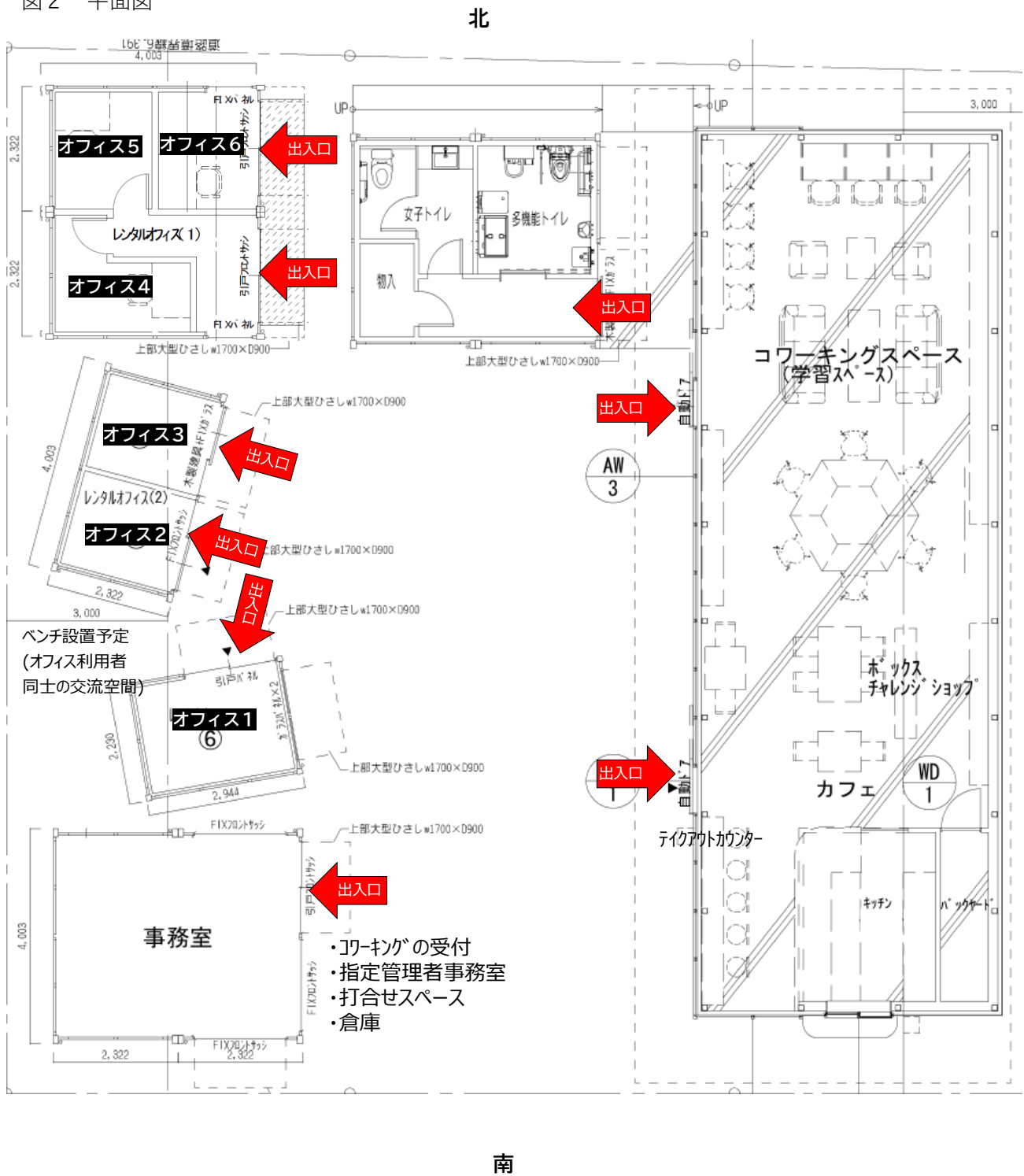
図2 平面図
